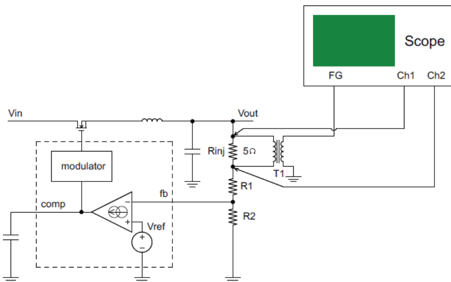
图 2: 环路响应测试时电源闭环反馈网络和示波器连接设置
